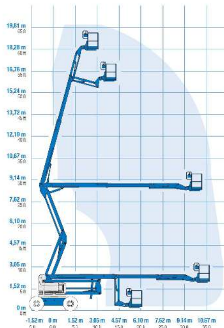
Arbeitsdiagramm Z-60/34
